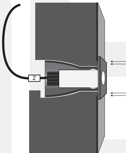
3.a Εφαρμογή στον τοίχο / Application in wall
