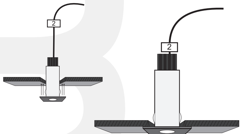
3.b Εφαρμογή στο ταβάνι / Application on ceiling
